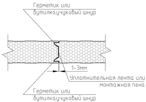
Рисунок 16. Стык стеновых панелей с замковым соединением Z-Lock
