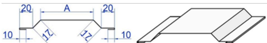
Рисунок 41. Фигурный нащельник
