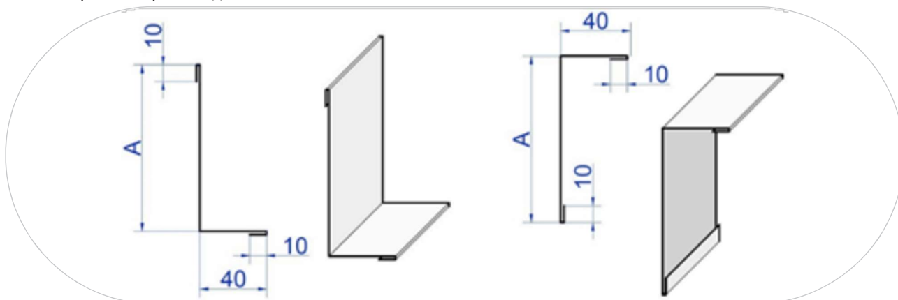
Рисунок 40. Уголки неравносторонние для стыков потолочных и стеновых панелей
